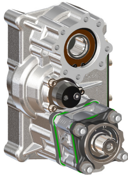
PTO Serien HIGH-POWER für ZF TRAXON Getrieben.
