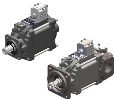
Axialkolben-verstellpumpen „PPV“.
