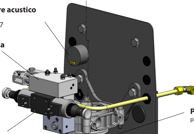
Staffa fissaggio Rear bracket 53800600200
