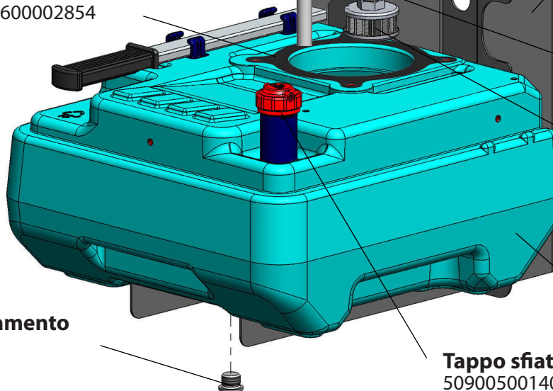
Guarnizione/Gasket 50600002854
