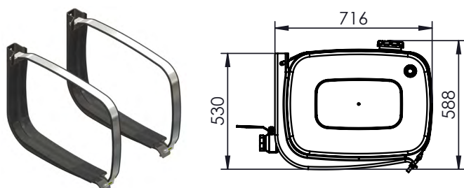
Montaggio laterale Side mounting
