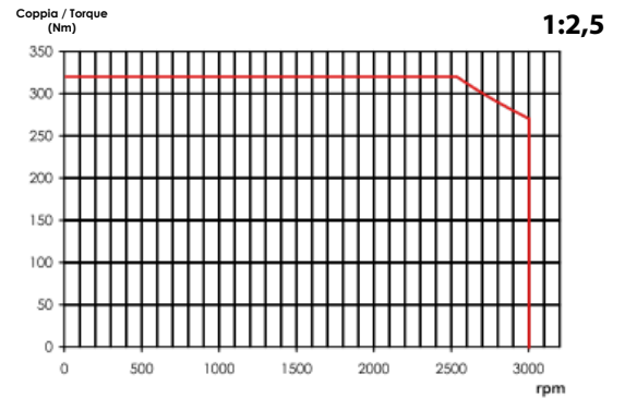
Coppia max. prelevabile USCITA Max. allowed torque OUTPUT
