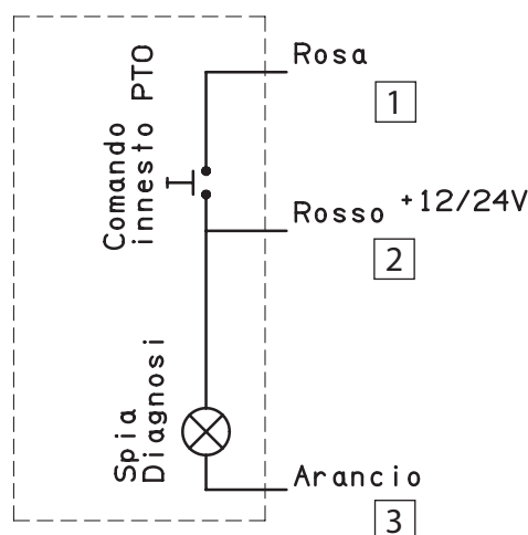
SCHEMA PULSANTE INNESTO PTO
