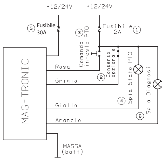
SCHEMA CABLAGGIO
